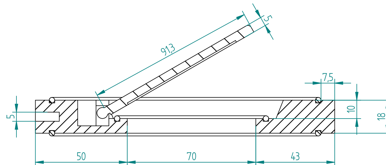
SECTION A-A
