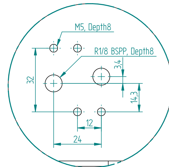
DETAIL A 1:1
