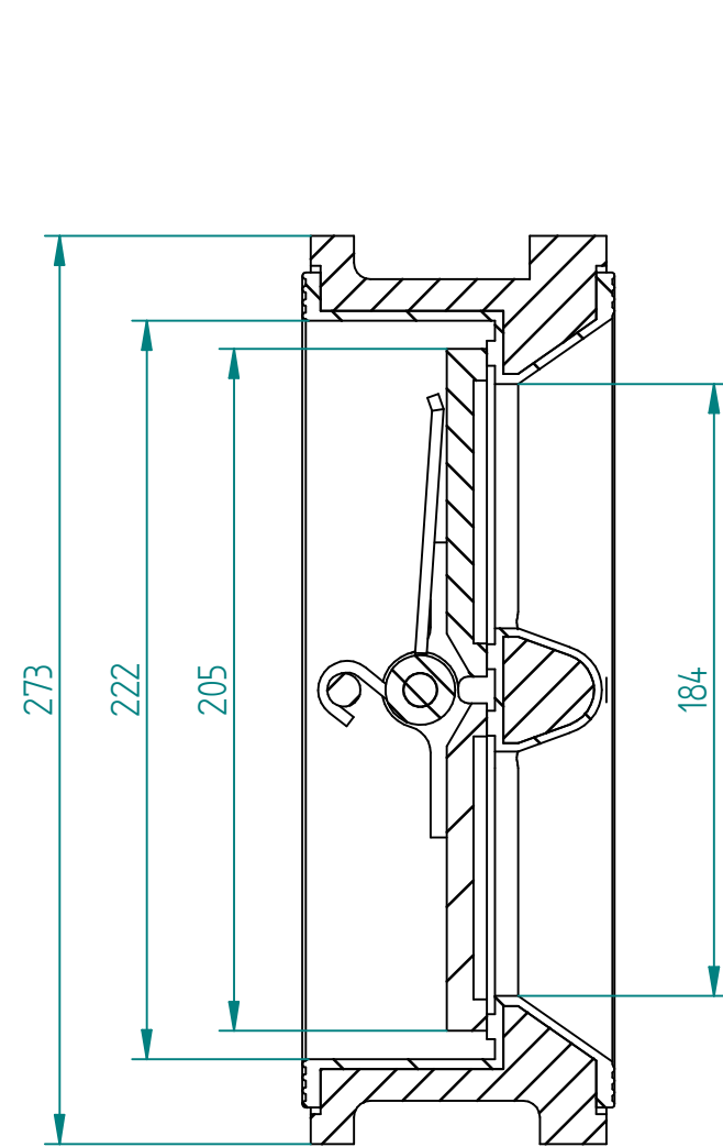
SECTION A-A
