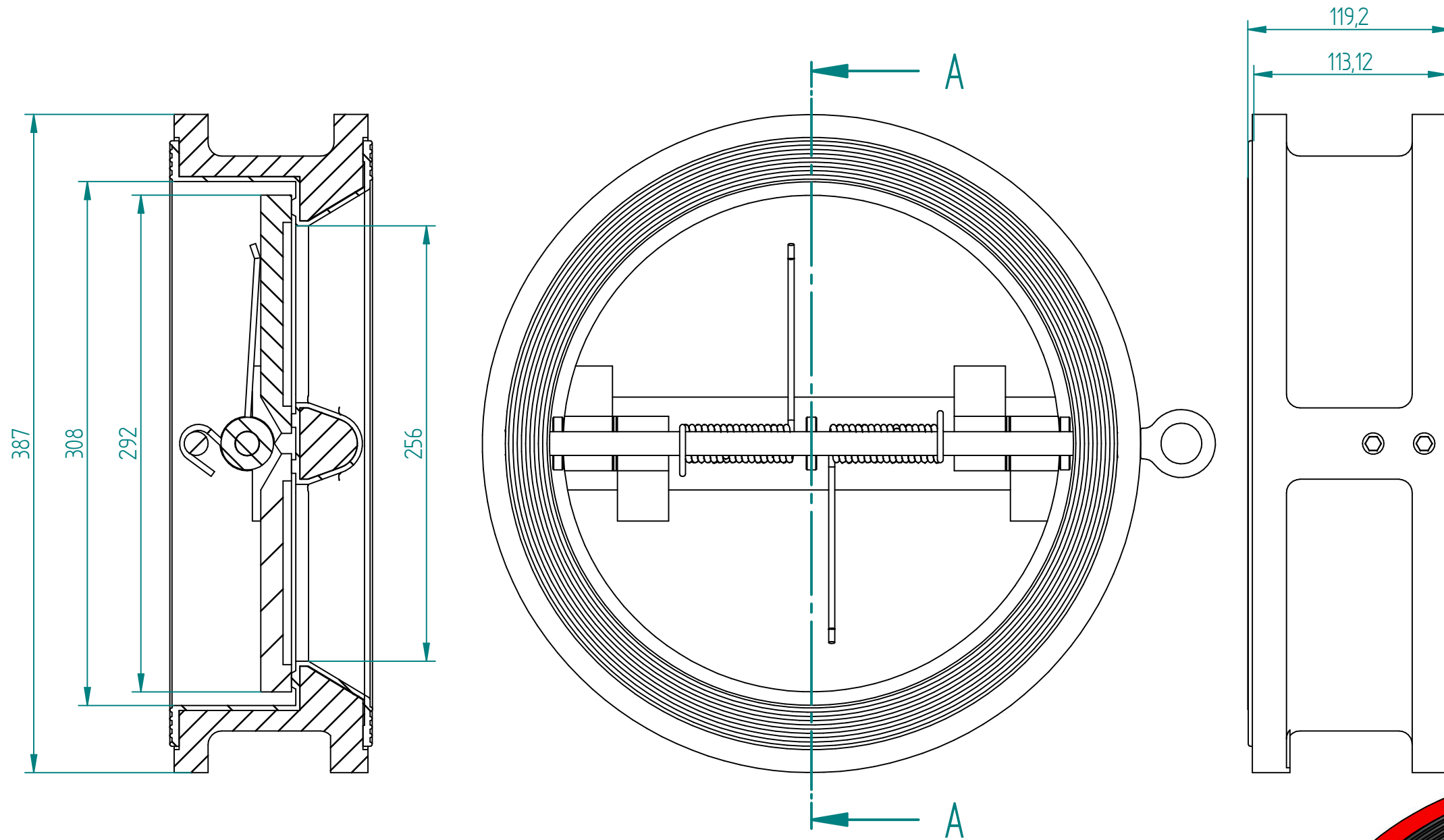
SECTION A-A
