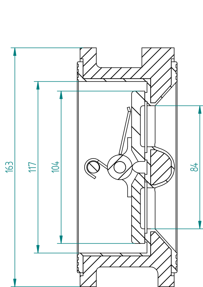
SECTION A-A
