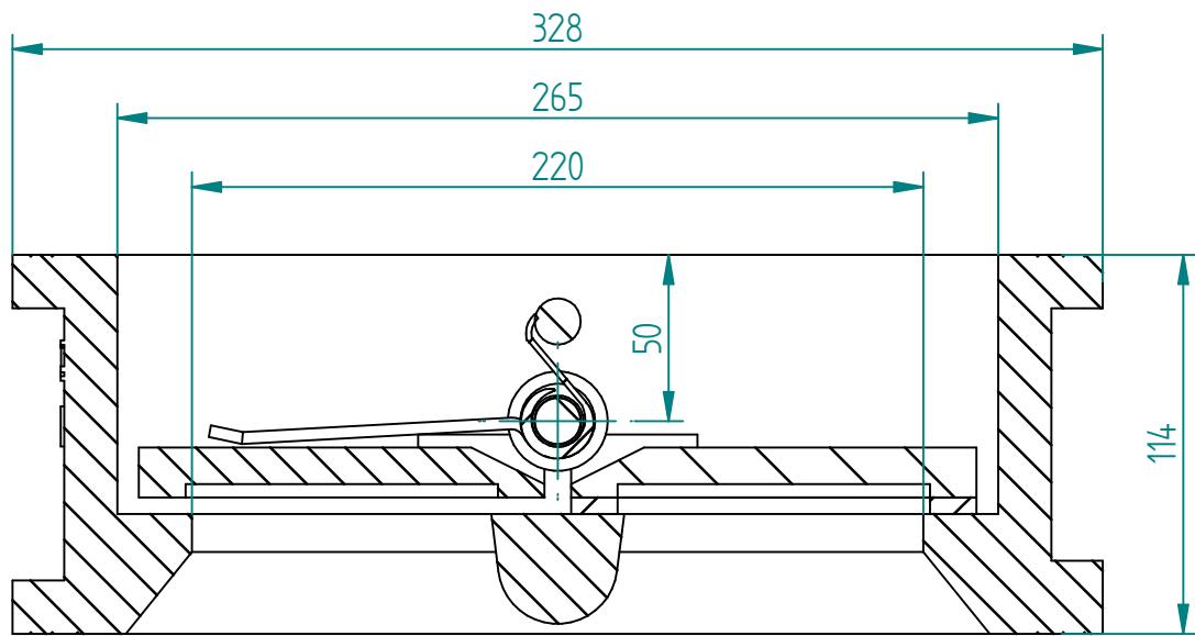
SECTION A-A
