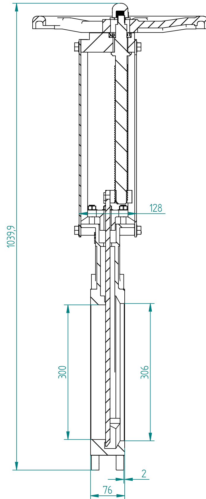
SECTION A-A
