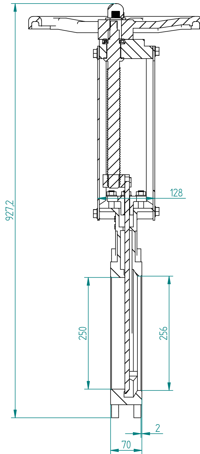
SECTION A-A
