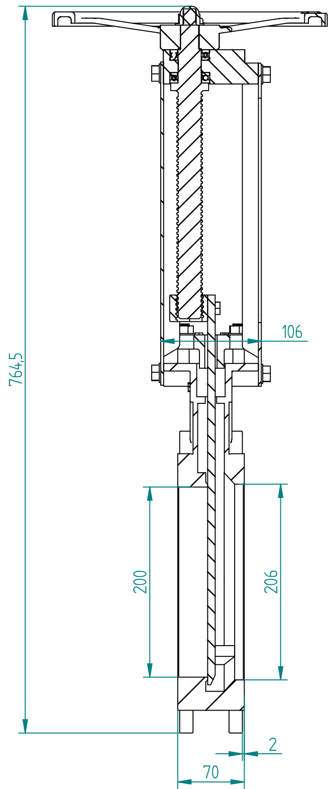
SECTION A-A
