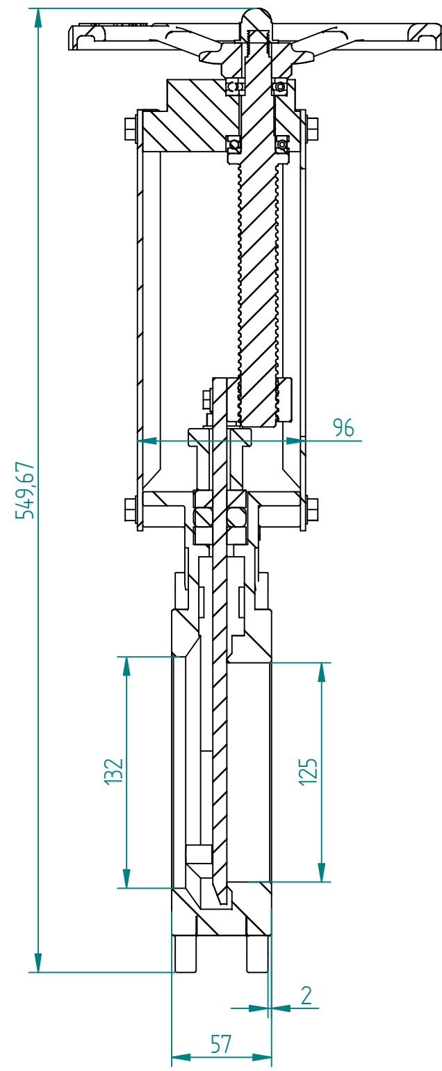
SECTION A-A
