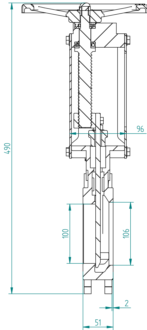
SECTION A-A
