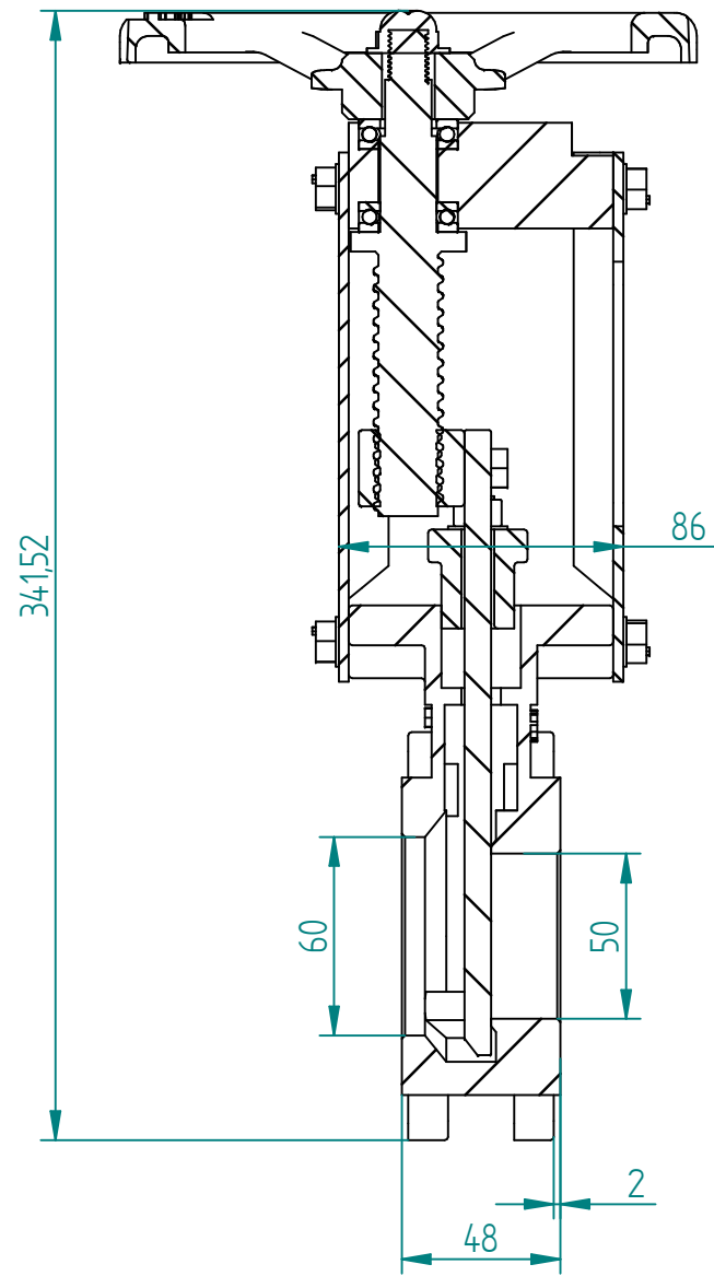
SECTION A-A
