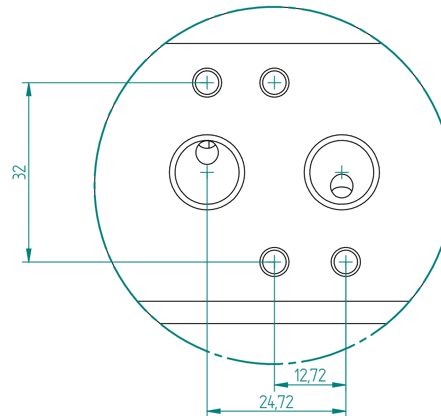
DETAIL A 1,5:1
