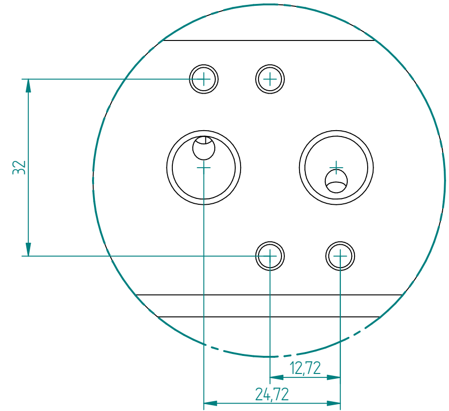
DETAIL A 1,5:1
