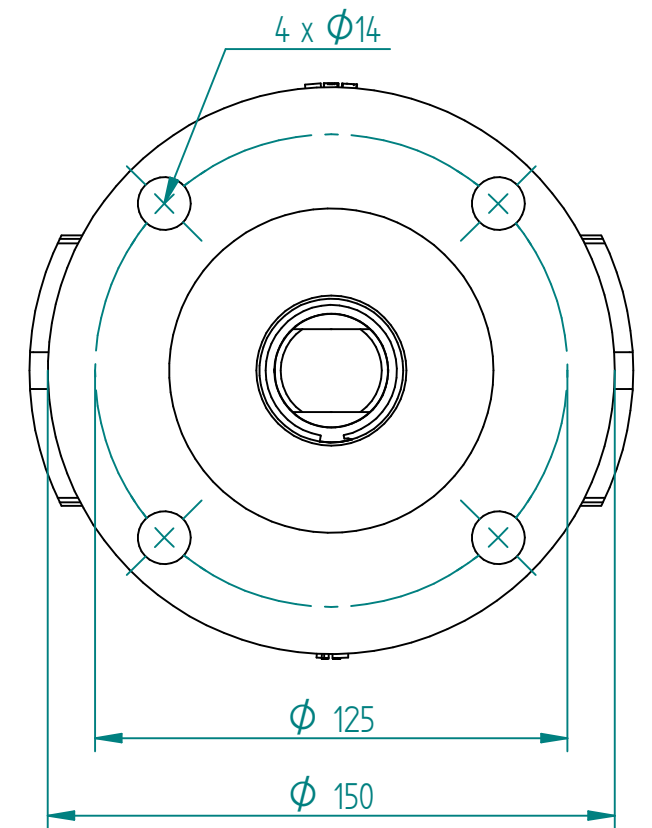
1:2 Top Plate
